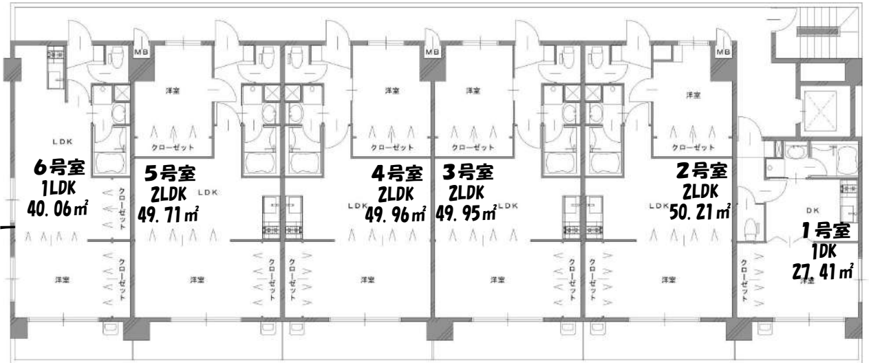
【2～7階平面図】
