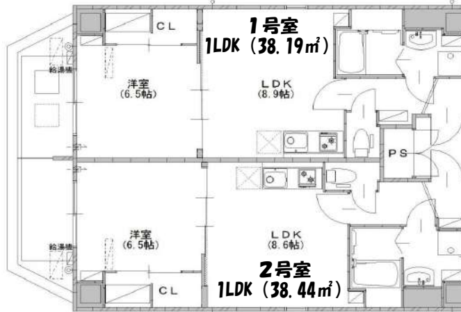
【2～8階平面図】
